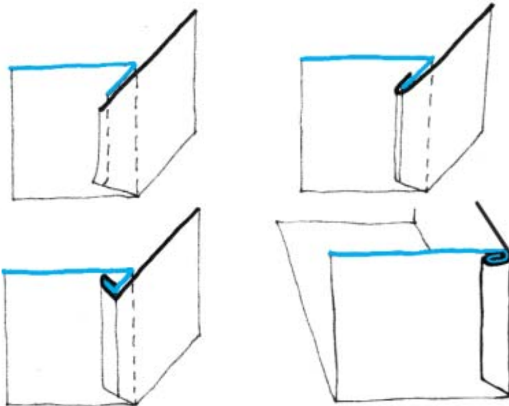
Attikacsatorna véglemezésének kialakítása
