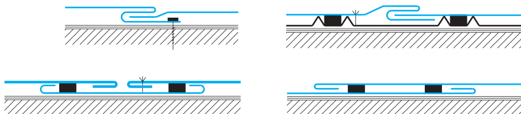
Speciális lemezcsatlakozások
