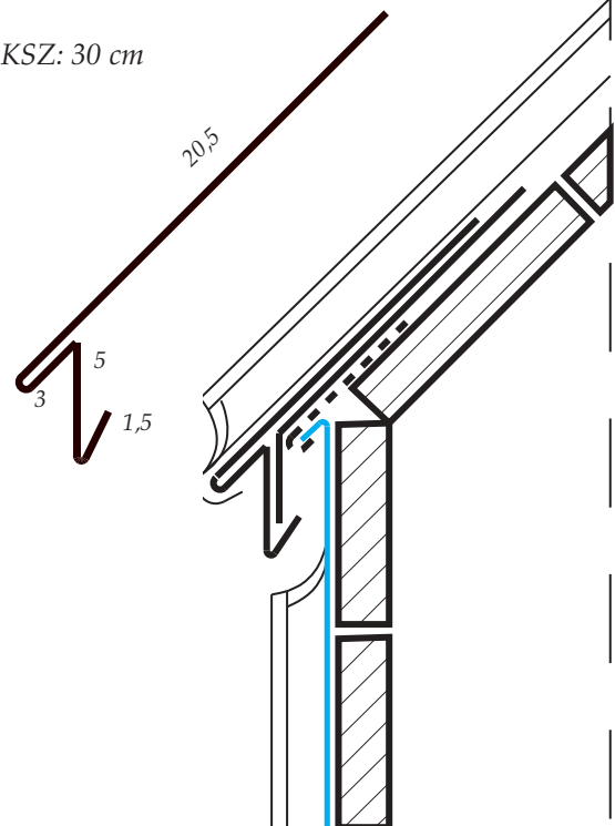
Korcolt tetővel történő zárt csatlakozásoknál a kiszellőzést más helyen kell megoldani.
