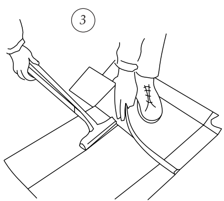
I. Attikacsatorna sarok kialakításának szabásterve és műveleti fázisai (finn korc)
