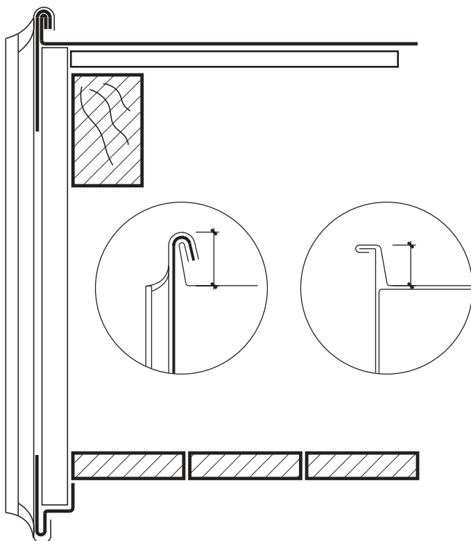
PLX Sávos homlokzati és tetőfedés oromcsatlakozása
