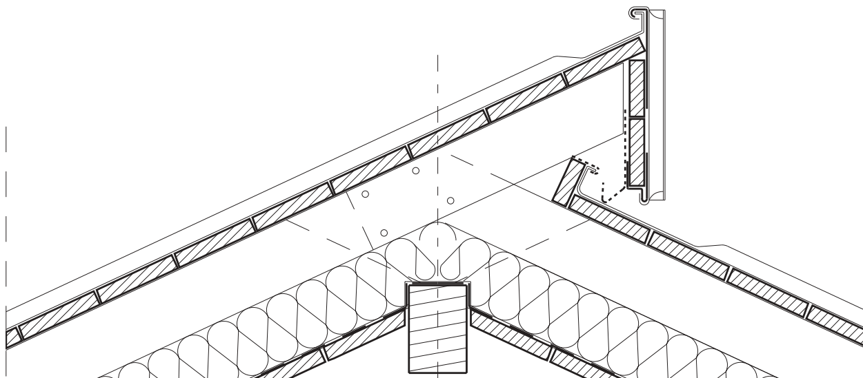
Egyoldali gerincszellőző
