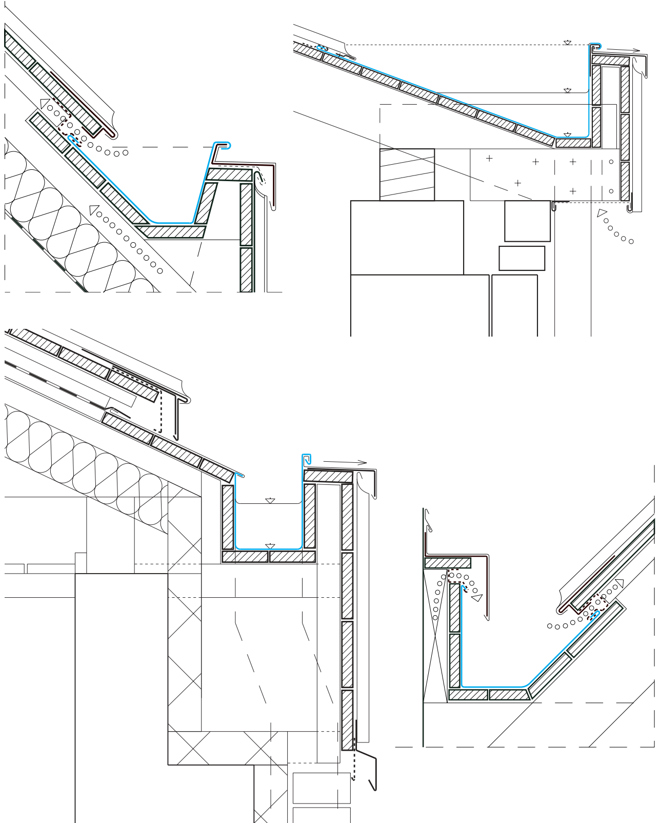
Attikacsatornás tetőszerkezet átszellőztetése
