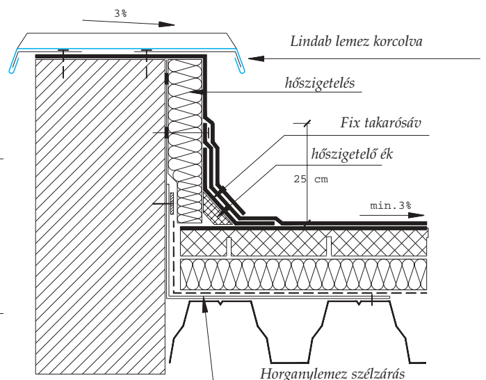
Attikafedés
