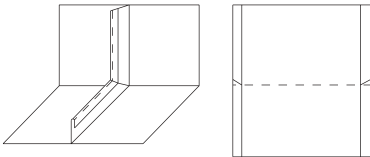
Gyűrt korcos felhajtás készítésének szabásterve
