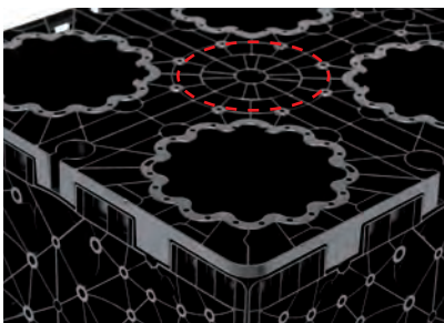
Vor dem Einbau der Grundelemente sind die Öffnungen für die Be- und Entlüftung bzw. die Inspektionsöffnungen am Grundelement auszuschneiden!
