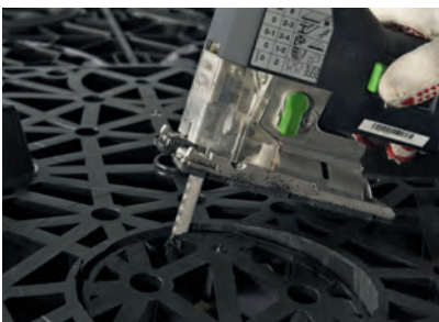
Aussägen der Rohranschlussadapteröffnung an der Seitenwand
