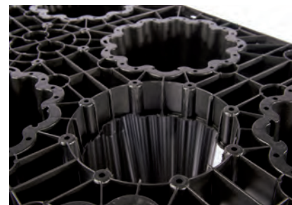
Vor dem Einbau der Grundelemente sind die Öffnungen für die Be- und Entlüftung bzw. die Inspektionsöffnungen am Grundelement auszuschneiden!
